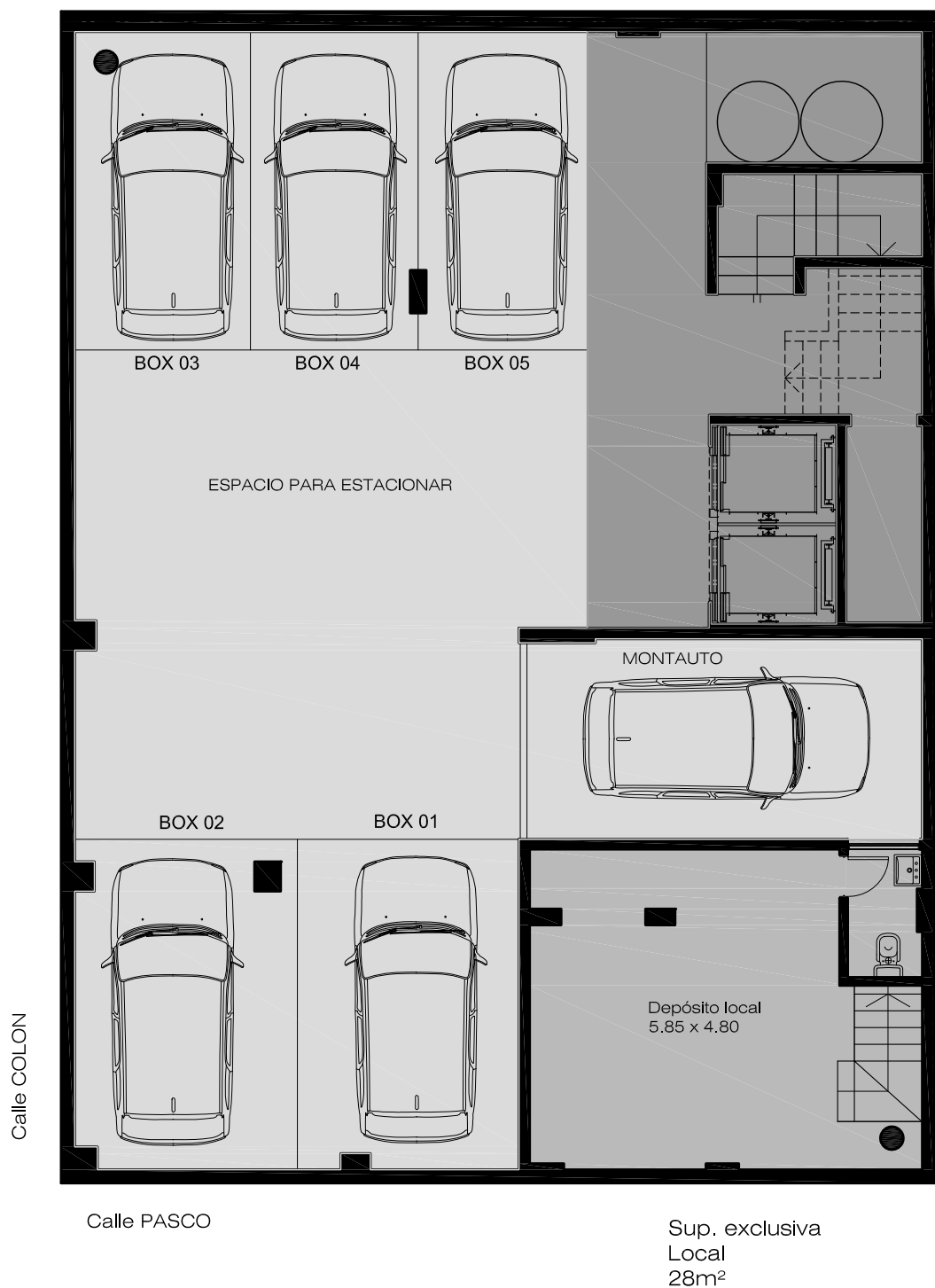
PLANTA SUBSUELO · COCHERA
